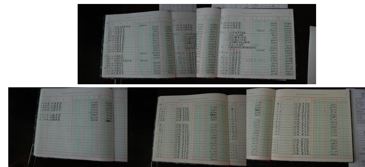
图 15 现金流水账
