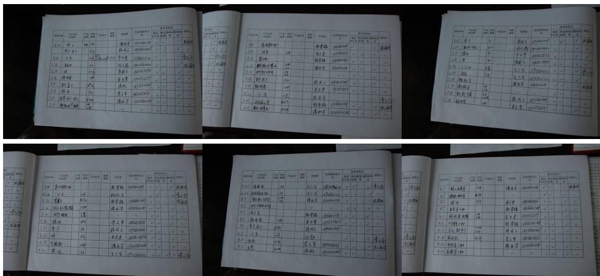
图 13 入库登记
